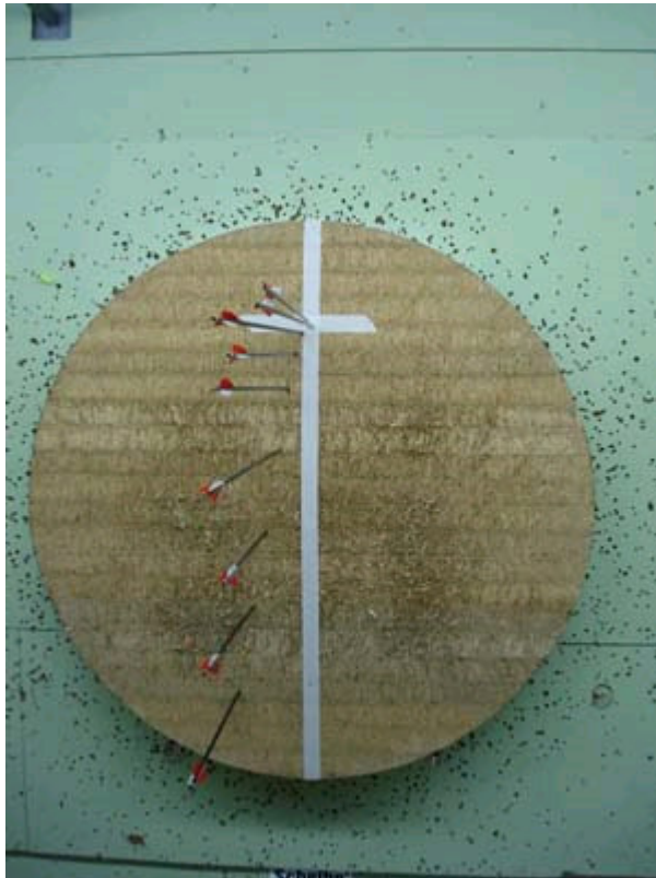
Bild 3: Button-Druck zu hoch Lineare Ablenkung nach links Botten-Druck herabsetzen
