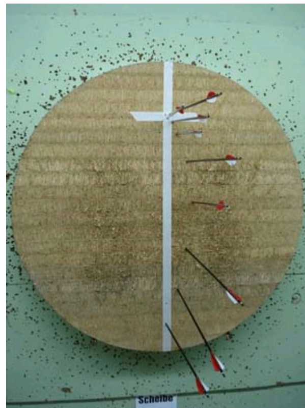
Bild 2: Button zu wenig im Bogenfenster Bauch nach rechts Button zum Pfeil hin aus dem Bogenfenster
